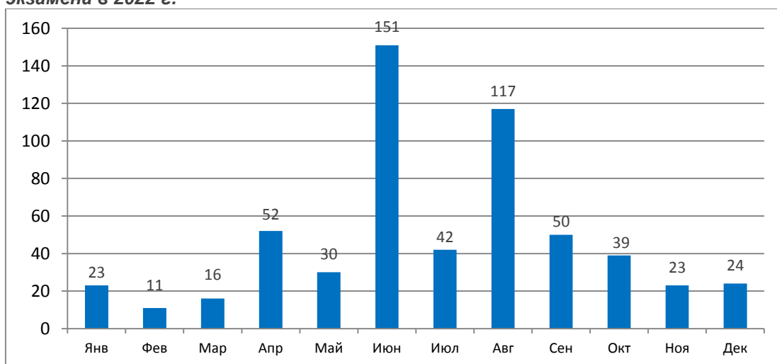
Рис. 1. Динамика первичных регистраций претендентов на сдачу модульного экзамена в 2022 г.
